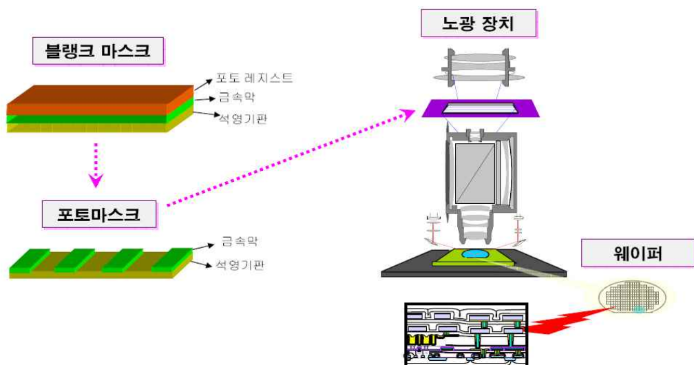
< 블랭크 마스크, 포토마스크 및 웨이퍼와의 관계 >
